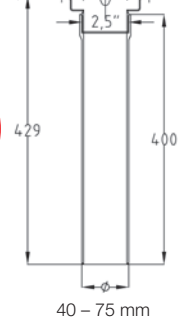
Capacità di scarico QS-M-75-400, per coperture in membrana
