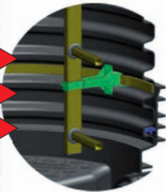
Foto 4. Dettaglio – staffe posizionate sull'anello di sostegno
