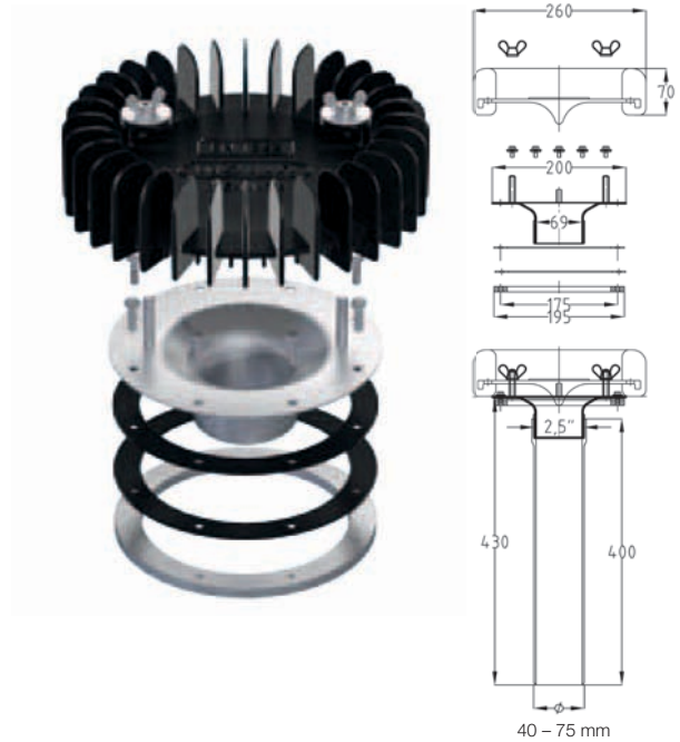
Capacità di scarico ricettore QS-M-75-260, per canale di gronda
