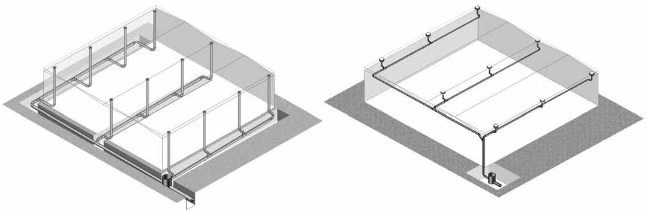
Figura 5. Esempio di sistema di drenaggio tradizionale (a sinistra) e di sistema di drenaggio sifonico (a destra).
